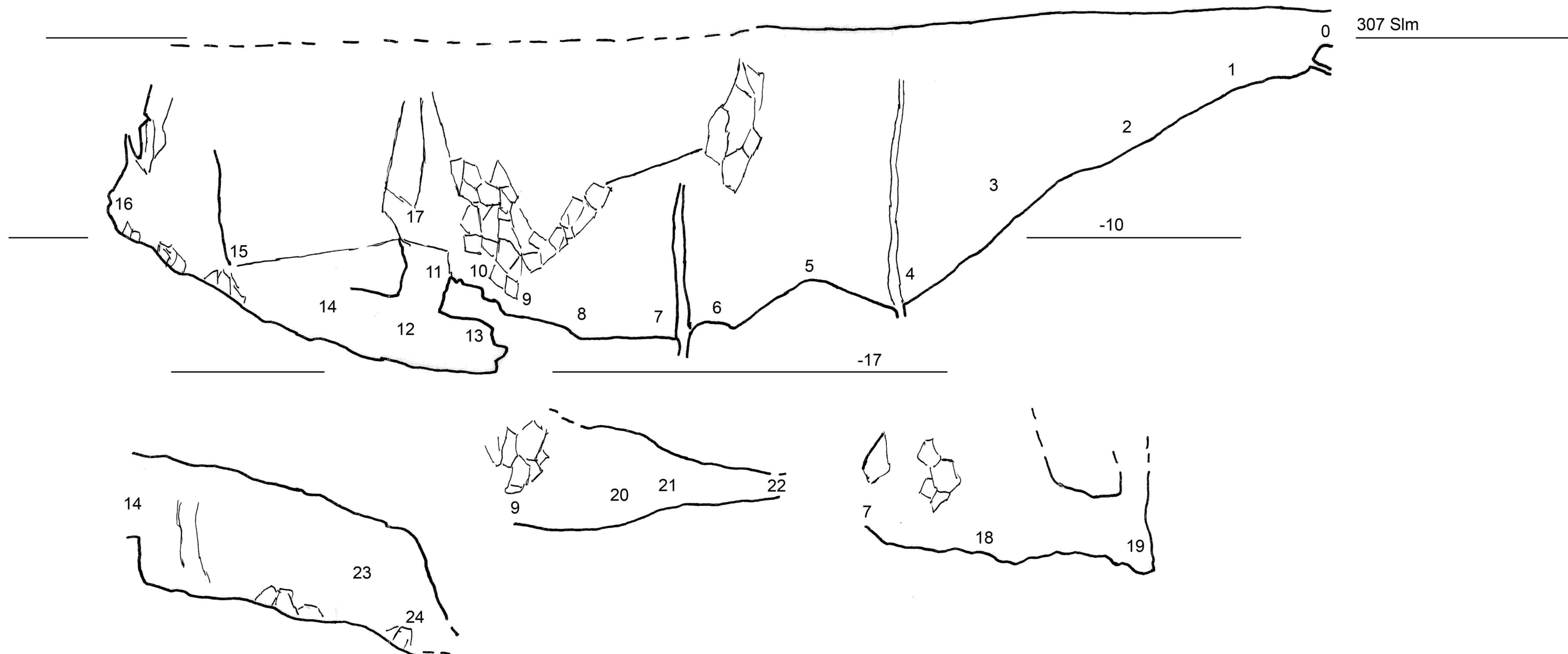
Sezione Longitudinale
